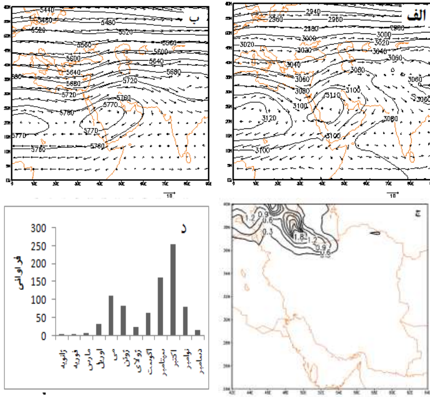
شکل ۵- (الف) میانگین روزانه ارتفاع ژئوپتانسیل و باد در تراز ۷۰۰؛ (ب) میانگین روزانه ارتفاع ژئوپتانسیل و باد تراز ۵۰۰ هکتوپاسکال؛ (ج) میانگین روزانه بارش (میلی‌متر در روز)؛ (د) فراوانی ماهانه رخداد الگوی چهارم
