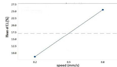
شکل ۱۷ - اثر فاکتور اصلی جنس بر ازدیاد طول
