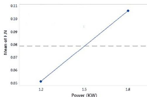
شکل ۳ - اثر توان بر عدد فریت
