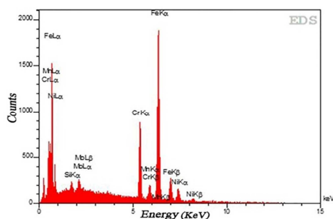
شکل ۲۲ - آنالیز عنصری نمونه 3B
