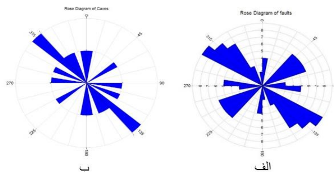
شکل (۴) الف - نمودار گلسرخی امتداد گسل‌های منطقه ب - نمودار گلسرخی امتداد غارهای منطقه
