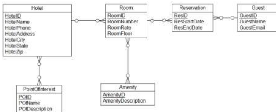
شکل ۷: مدل مفهومی سیستم رزرو هتل
