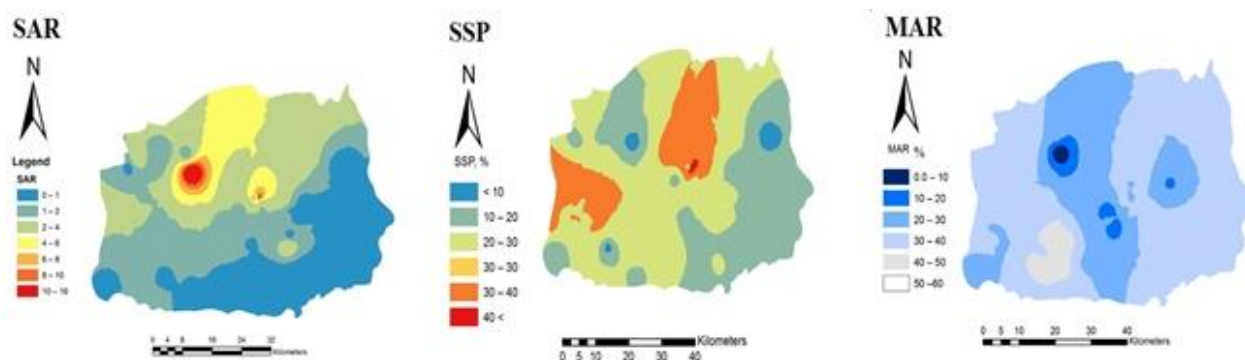
شکل ۱۰- نقشه هم ارزش مقادیر SAR، SSP و MAR.
