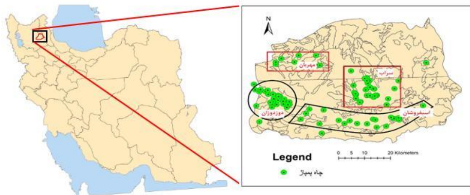
شکل ۲- موقعیت جغرافیایی چاه‌های پمپاژ و حدود آبخوان‌های منطقه مورد مطالعه. جدول ۱- مقایسه بیشینه مجاز غلظت عناصر در آب آبیاری.
