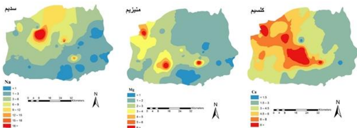
شکل ۶- نقشه هم ارزش سدیم، کلسیم و منیزیم در دشت سراب.
