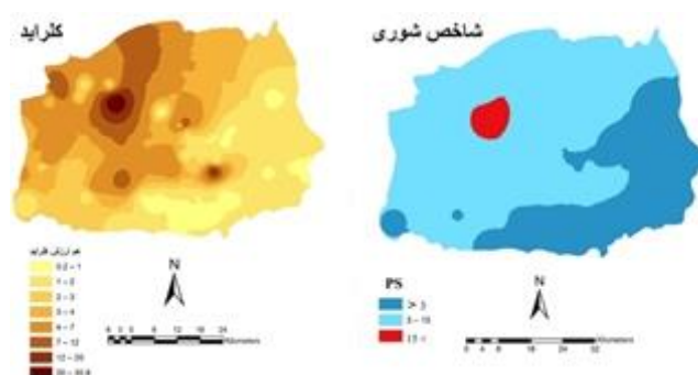
شکل ۵- تغییرات مکانی کلراید و شاخص پتانسیل شوری در دشت سراب.
