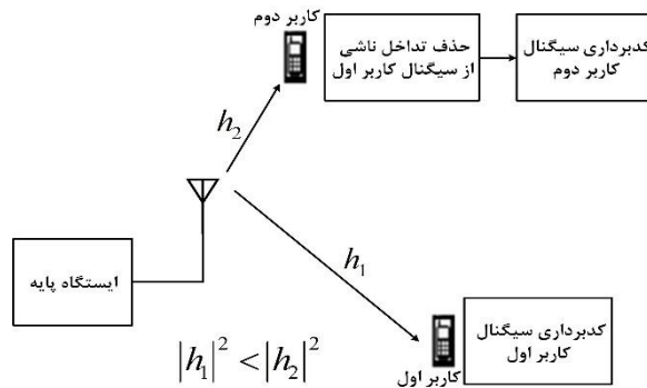
شکل ۱: یک سیستم NOMA با یک ایستگاه پایه و ۲ کاربر در لینک فروسو
