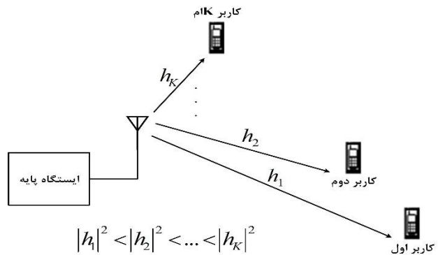
شکل ۲: یک سیستم NOMA با یک ایستگاه پایه و K کاربر در لینک فروسو
