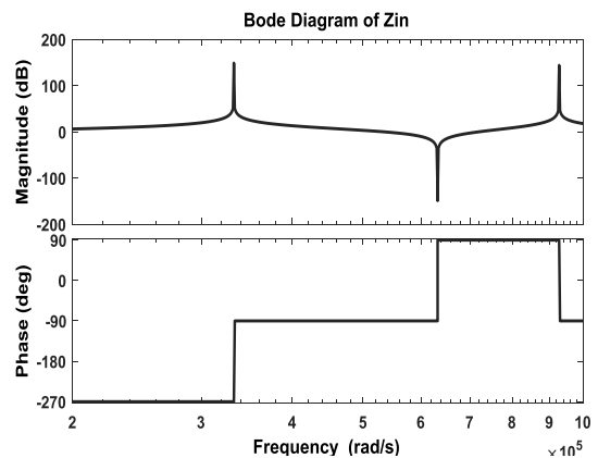
شکل ۴: پاسخ فرکانسی امپدانس ورودی مبدل
