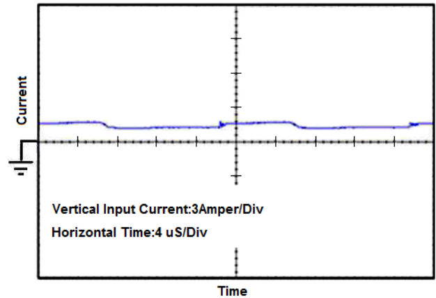
شکل ۱۴: شکل موج جریان ورودی مبدل به ازای P_o=45W
