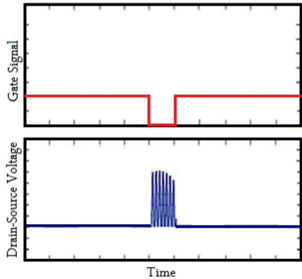
شکل ۷: صفر شدن متناوب ولتاژ درین-سورس ماسفت در مبدل پیشنهادی در هنگام عدم وجود فرمان گیت
