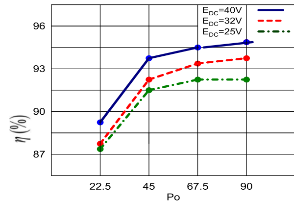
شکل ۱۷: منحنی تغییرات بازده با تغییر توان بار در ولتاژهای ورودی مختلف شبیه سازی در دو حالت انجام می گیرد. حالت اول؛ سیکل کاری مبدل ثابت در نظر گرفته می شود ( D=0.7 ) برای این منظور کلید ورودی مولد PWM شکل ۱۸ در وضعیت ۱ قرار داده می شود. در این شرایط تغییرات ولتاژ آرایه فتوولتاییک با نسبت بهره مبدل به خروجی هم منتقل می شود. شبیه سازی به ازای مقاومت بار ۱۲۰۰ اهم انجام شده است.
