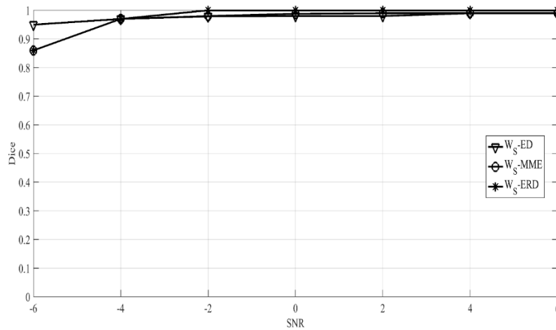
شکل ۹: مقایسه عملکرد همزمان‌سازی برای طول‌های برست کوتاه بر روی آشکارسازهای مختلف
