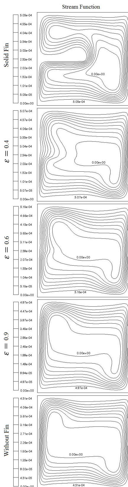
شكل ٨- خطوط جریان، پره متخلخل با میزان تخلخل‌های مختلف ( Ra = 10^4 و Da = 10^{-2} ، \alpha = 90^\circ ، S = 0.5 ، L = 0.5 )
