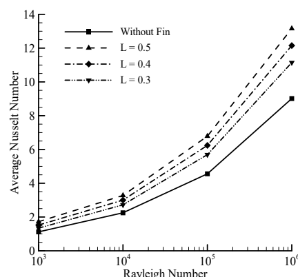
شکل ۵- تاثیر طول پره متخلخل بر عدد نوسلت در اعداد رایلی
