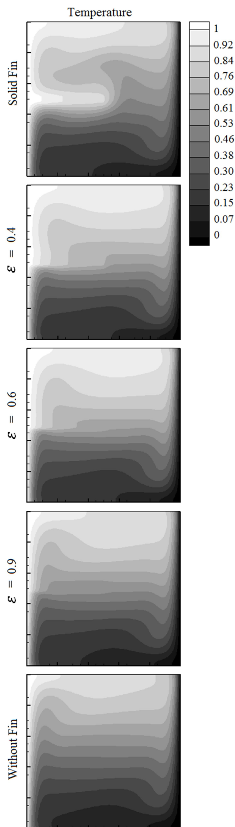
شكل ٩- خطوط همدمای پره متخلخل با میزان تخلخل‌های مختلف ( Ra = 10^4 و Da = 10^{-2} ، \alpha = 90^\circ ، S = 0.5 ، L = 0.5 )
