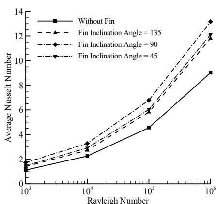
شکل ۶- تاثیر زاویه نصب پره متخلخل روی دیواره گرم بر عدد نوسلت در اعداد رایلی مختلف ( \varepsilon = 0.9 , S = 0.5 , L = 0.5 ) و
