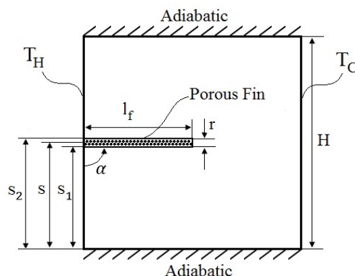
شکل ۱- هندسه مورد مطالعه
