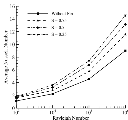
شکل ۴- تاثیر محل نصب پره متخلخل روی دیواره گرم بر عدد نوسلت در اعداد رایلی مختلف ( \varepsilon = 0.9 , \alpha = 90^\circ , L = 0.5 ) و
