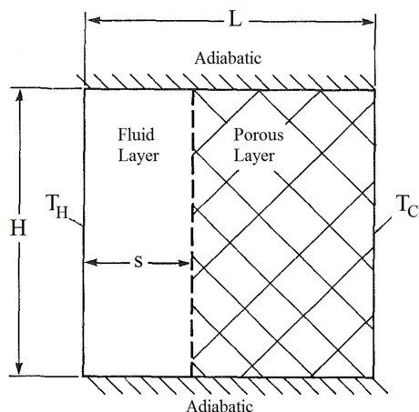
شکل ۲- شکل طرحواره سیستم مورد مطالعه بکرمین [۱۵]
