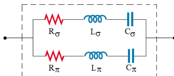
شکل 2: مدار الکتریکی معادل برای گرافین با رسانندگی تعریف شده
