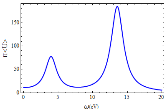
شکل 3: نمودار چگالی انرژی الکتریکی در گرافین با رسانندگی
