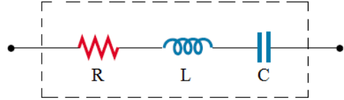
شکل ۱: مدار الکتریکی معادل برای گرافین با رسانندگی تعریف شده در رابطه (۳)
