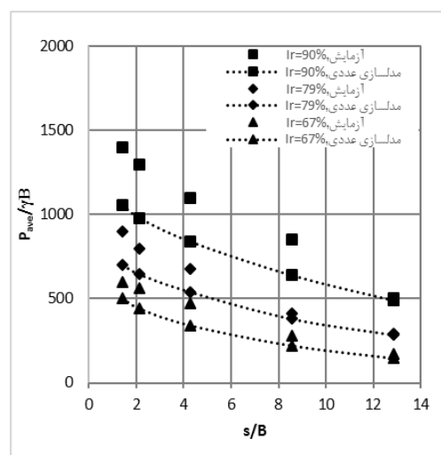
شکل ۳- مقایسه روش مدل‌سازی عددی و نتایج آزمایشگاهی برای نمودار نسبت p_{ave}/\gamma B در مقابل s/B
