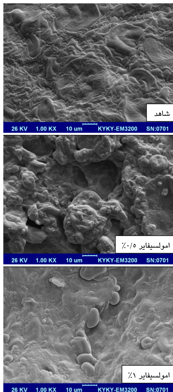
شکل ۵- تصاویر میکروسکوپ الکترونی روبشی (SEM) نمونه‌های حاوی امولسیفایر و یا آنزیم در بزرگنمایی ۱۰۰۰
