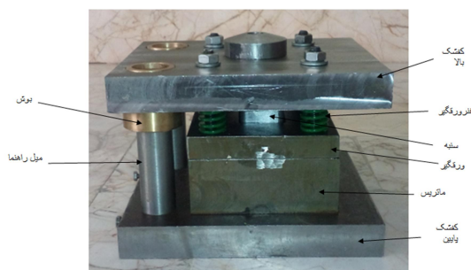
شکل ۱۳- قالب کشش
