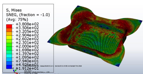
شکل ۶- کانتور تنش ون میزز
