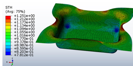
شکل ۸- کانتور تغییرات ضخامت
