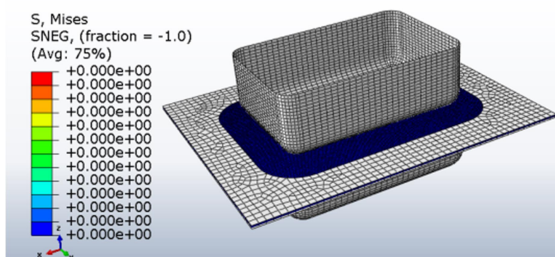
شکل ۴- قالب شبیه سازی شده در شروع عملیات کشش
