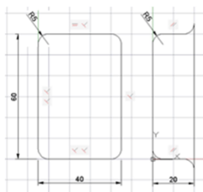
شکل ۳- ابعاد ورق شبیه سازی شده
