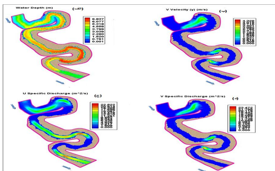
شکل (۶) پارامترهای عمق آب (الف)، سرعت در راستای عرضی (ب)، دبی ویژه در راستای طولی (ج) و عرضی (د) رودخانه برای دبی با دوره‌ی بازگشت ۵۰ سال
