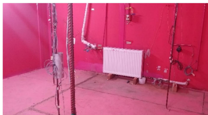
شکل ۲- رادیاتور پانلی در حین آزمون
