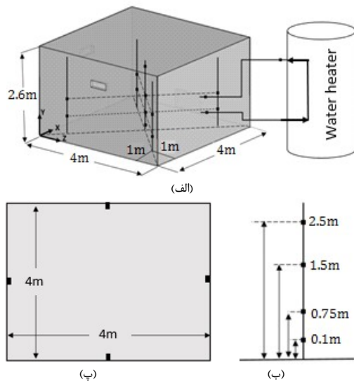
شکل ۱- اتاق آزمون (الف) - اتاق آزمون. ب- دماسنج های عمودی وسط اتاق. پ- نما از بالا
