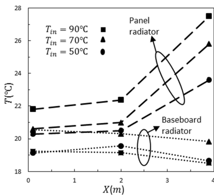
شکل ۵- توزیع دما در صفحه (Y = 1.5 و Z = 2)
