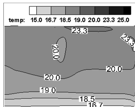
شکل ۱۶- توزیع دمای عددی در صفحه تقارن اتاق ( X=2 ) برای رادیاتور پانلی
