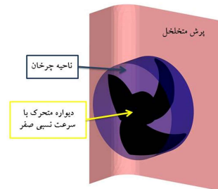
شکل ۶- شرایط مرزی حل جریان، فضای محاسباتی (ب) ناحیه چرخان، فن جریان محوری و مبادله‌کن گرما
