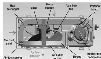
شکل ۱- نمایی از واحد بیرونی یک کولر گازی دو تکه با قسمت‌های مختلف آن [۱]
