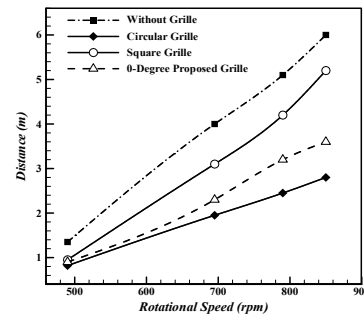
شکل ۱۵- پرتاب هوای فن بر حسب سرعت دورانی
