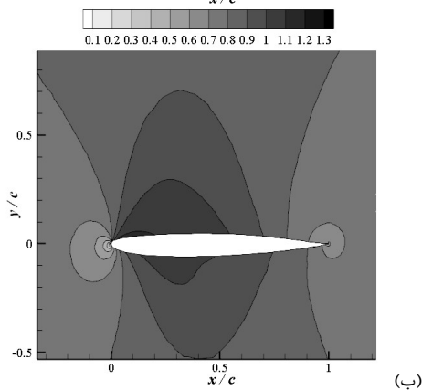
شکل ۷- کانتور عدد ماخ (الف) هندسه پایه (ب) نمونه A
