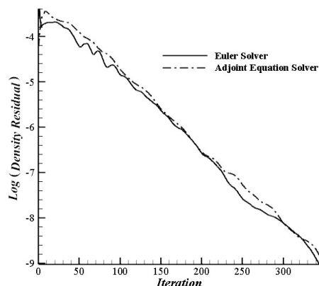
شکل ۶- روند همگرایی معادله اویلر و معادله الحاقی برای طرح اولیه نمونه A
