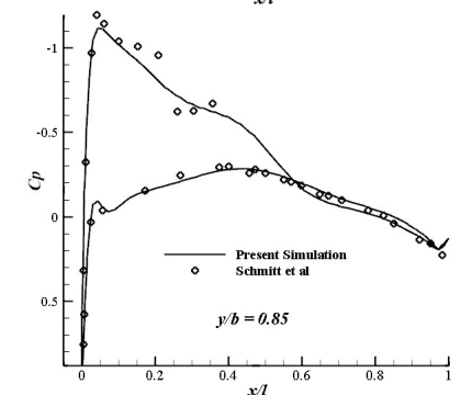
شکل ۳- ضریب فشار بر روی سطح ONERA M6 در سه مقطع مختلف در طول بال، مقایسه نتایج حاضر با داده های تجربی
