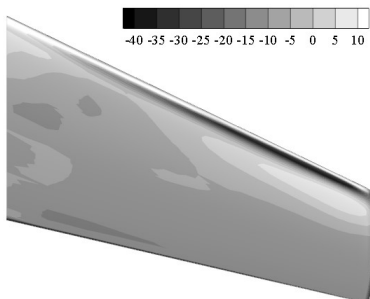
شکل ۱۰- کانتور حساسیت سطح نسبت به نیروی پسا
