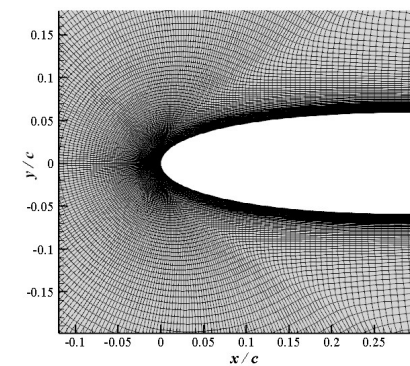
شکل ۴- شبکه محاسباتی اطراف دماغه ایرفویل NACA0012
