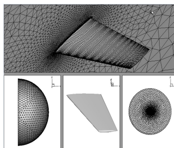
شکل ۲- سه نما از شبکه استفاده شده برای هندسه ONERA M6 همراه هندسه اصلی بال
