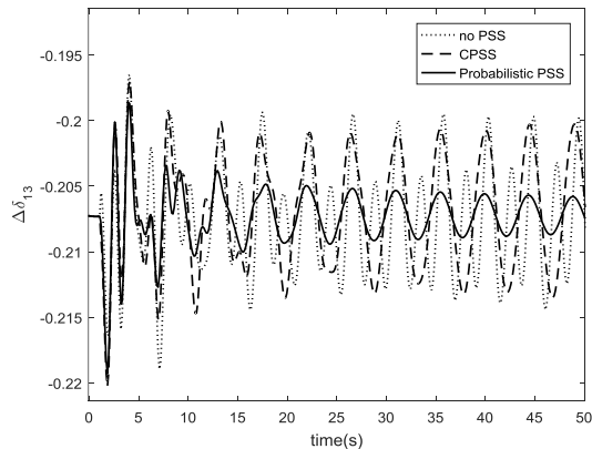
شکل ۸: اختلاف زاویه بین ماشین های ۱ و ۳ برای بار توان ثابت. (بار ۱/۸۵ برابری)
