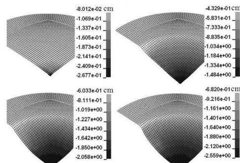
شکل ۱۶- تغییر شکل ورق طی فرایند شکل دهی الکتروهیدرولیکی
