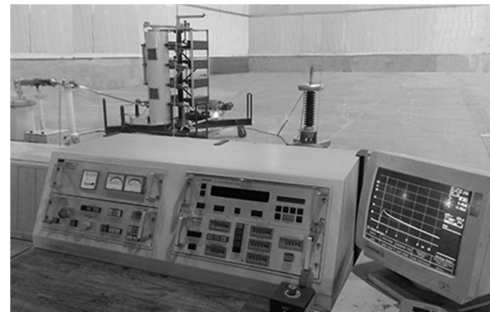
شکل ۲- تجهیزات فرایند شکل‌دهی الکتروهیدرولیکی
