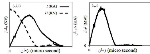
شکل ۱۱- نمونه‌های از نمودارهای به دست آمده برای (الف) جریان، ولتاژ (ب) توان الکتریکی
