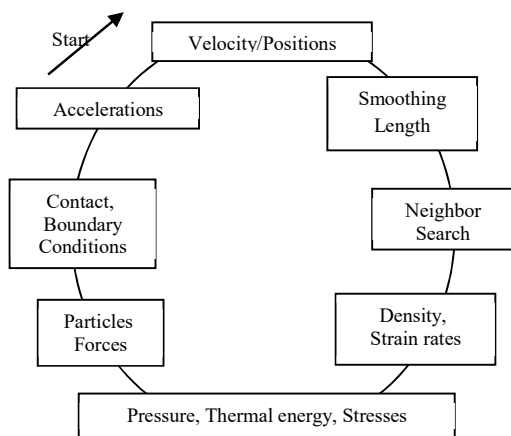
شکل ۷- روند محاسبات در روش هیدرویدینامیک ذرات هموار [۲۶]
