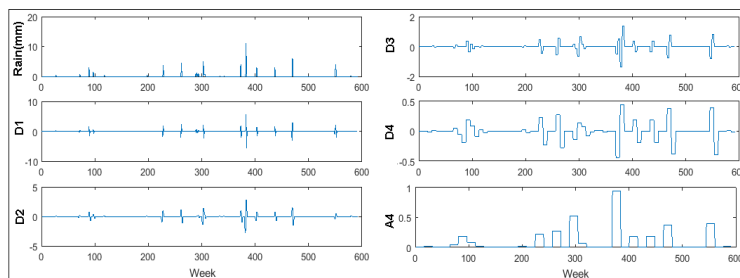
شکل ۷: تجزیه سیگنال بارش تابستانه بزم تا ۴ سطح
