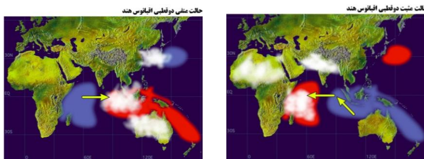
شکل ۲: فاز مثبت و فاز منفی پدیده دوقطبی اقیانوس هند (منبع: آژانس علم و تکنولوژی زمین - دریا ژاپن)
