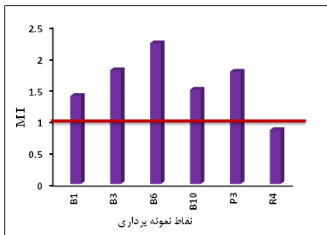
شکل ۱۳- تغییرات شاخص فلزی (MI) در تالاب برم‌شور.
