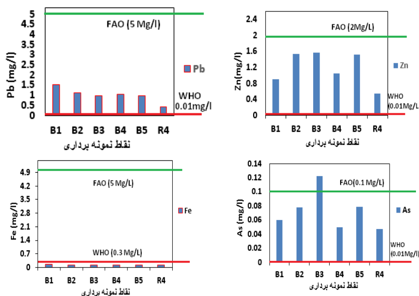
شکل ۱۲- غلظت فلزات سنگین و مقایسه با حد مجاز آبیاری (FAO) و سازمان بهداشت جهانی (WHO)
