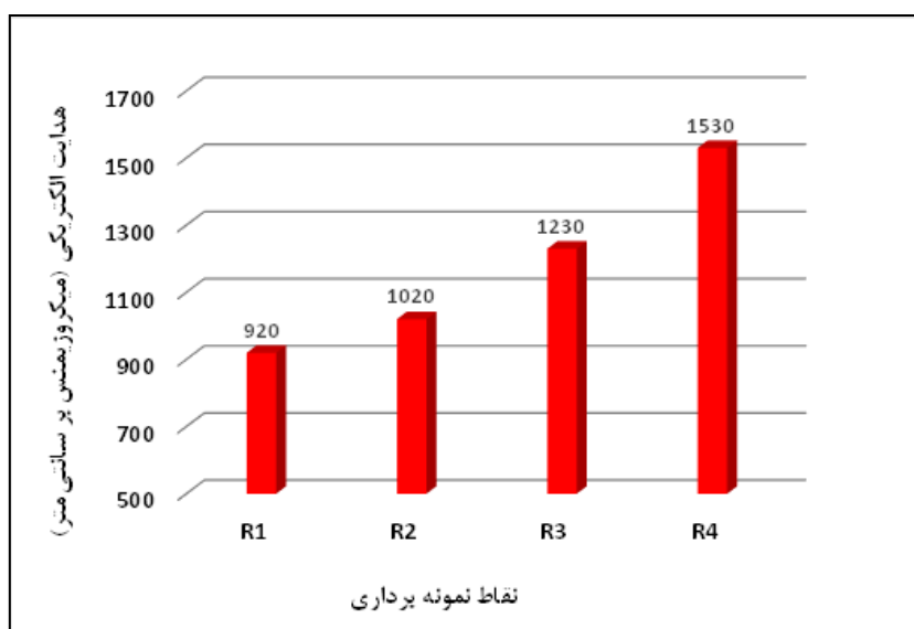
شکل ۴- تغییرات EC در آبراهه فصلی ورودی به تالاب از ارتفاعات سازند گچساران
