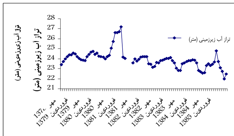
شکل (۶) نوسانات سطح آب زیرزمینی منطقه ائل‌گلی دشت تبریز (۱۳۷۸-۸۵)
