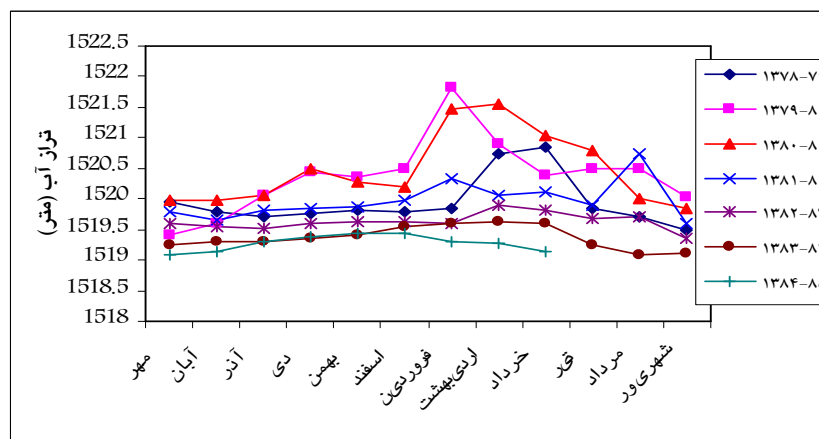
شکل (۹) نوسانات ماهانه و فصلی سطح آب زیرزمینی بارنج در دشت تبریز (۱۳۷۸-۸۵)
