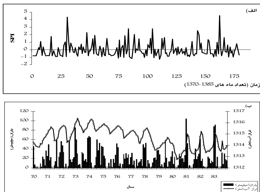
شکل (۱۰) نمودار مقادیر شاخص SPI (الف)، هیدروگراف تراز آب زیرزمینی و مقادیر بارش ماهانه (ب) در دوره آماری ۱۳۸۳-۱۳۷۰
