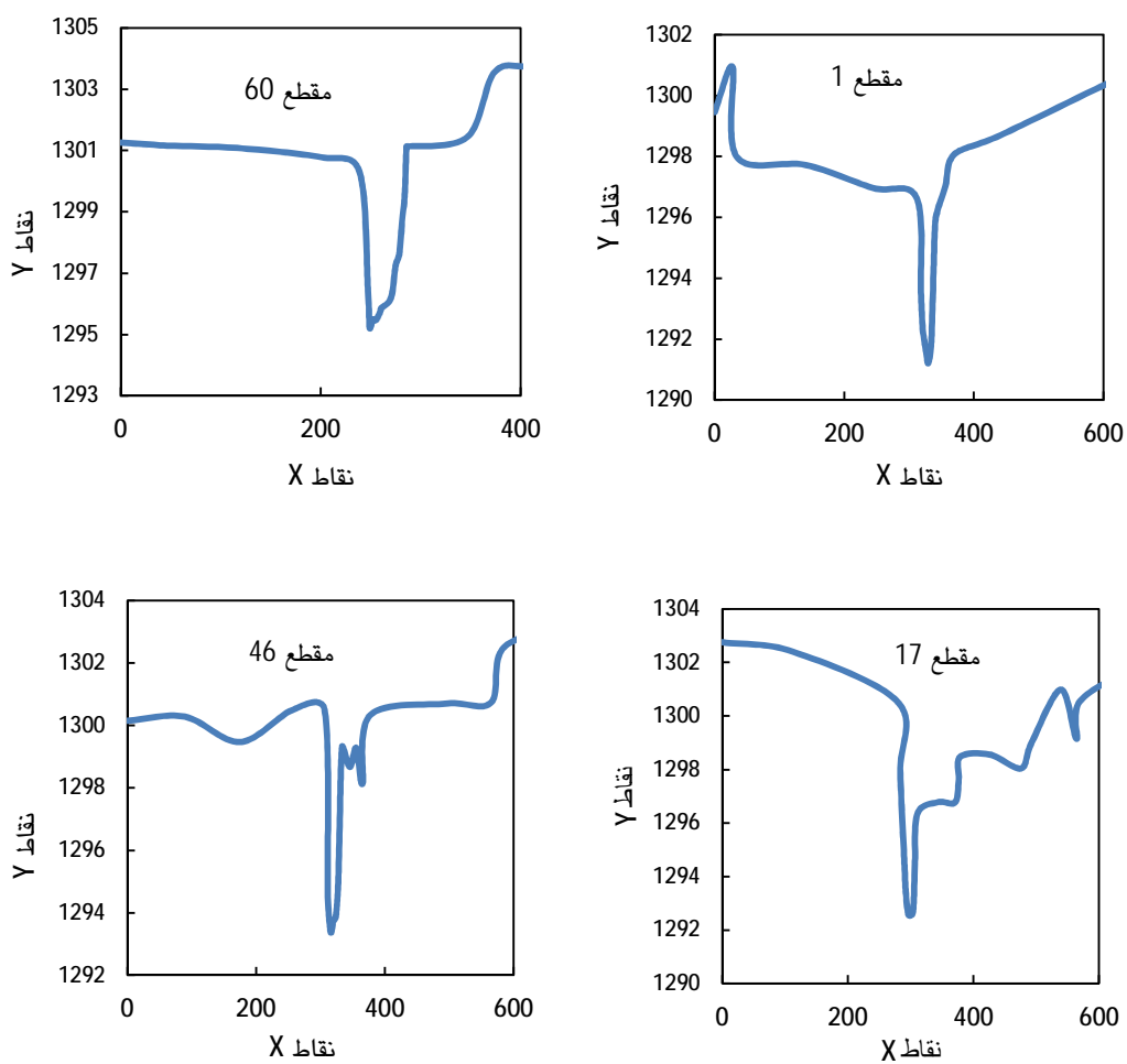
شکل 2- نیم‌رخ عرضی برخی مقاطع طبیعی رودخانه.
