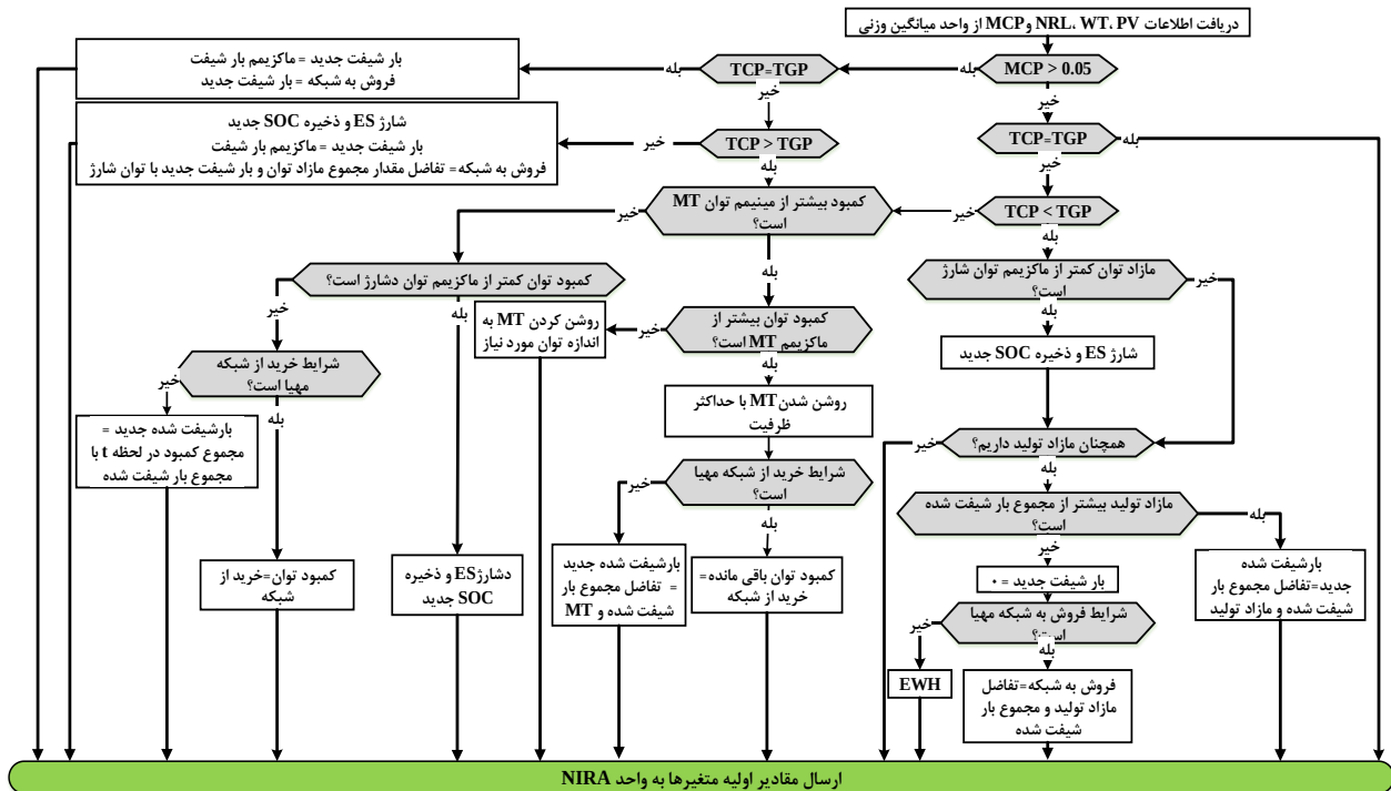
شکل ۵: فلوچارت پیاده‌سازی شده برای مدل‌سازی RLD
