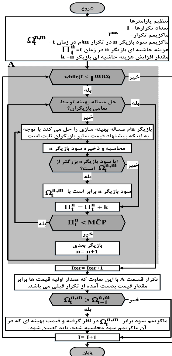
شکل ۷: واحد BSCG
