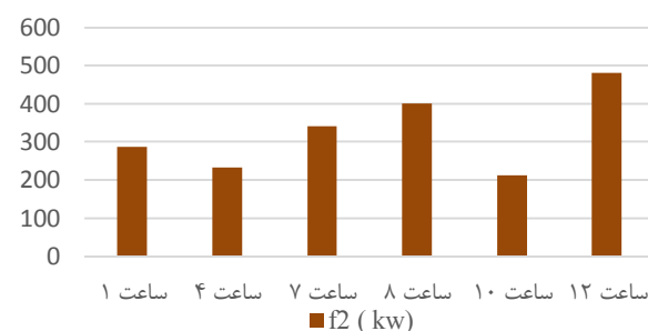
شکل ۹ - مقایسه توابع هدف به ازای عملکرد منابع در حالت کار با قیمت یکپارچه شبکه نسبت به عدم تزریق توان راکتیو
