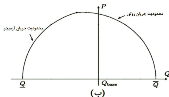
شکل ۶: منحنی قابلیت تزریق توان راکتیو؛ الف) ژنراتور سنکرون، ب) DFIG
