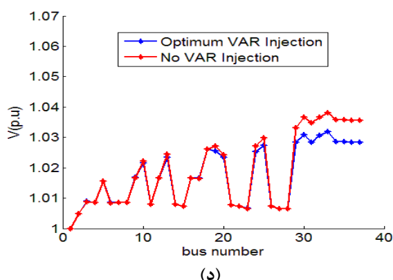
شکل ۱۰: مقایسه ولتاژ شبکه به ازای عملکرد منابع در حالت کار با قیمت یکپارچه نسبت به عدم تزریق توان راکتیو؛ (الف) ساعت ۱، (ب) ساعت ۴، (ج) ساعت ۸، (د) ساعت ۱۲
