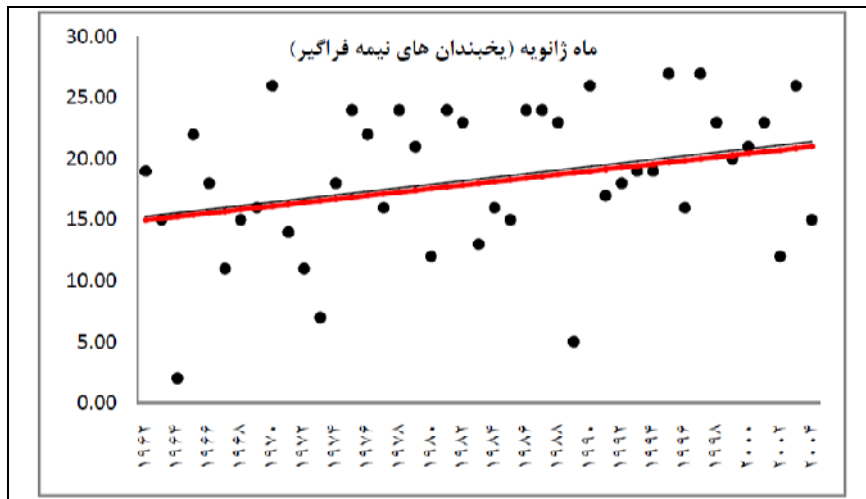
شکل (۵) نمودار روند تغییرات روزهای همراه با یخبندان‌های نیمه‌فراگیر ماه ژانویه ایران. خط قرمز پرنس برآورد تخمینگر شیب سنس و خط سیاه نازک برآورد در گرسبون خطی
