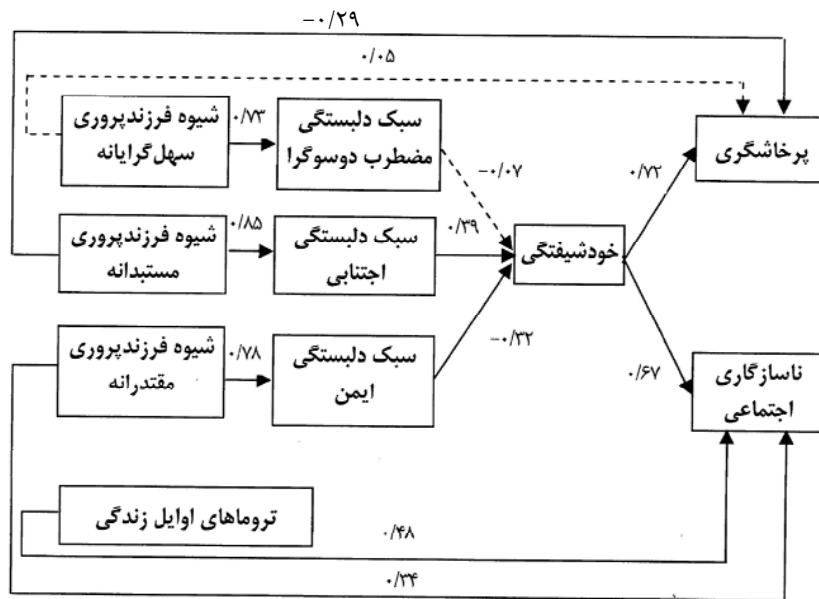
شکل (۲) الگوی نهایی در پژوهش حاضر به همراه ضرایب استاندارد مسیره‌ها و مسیره‌های حذف شده
