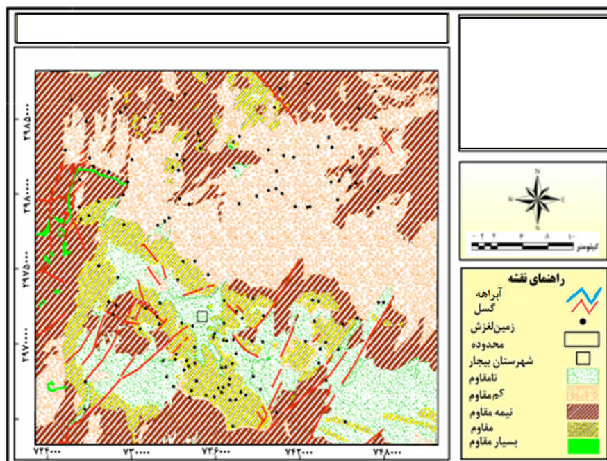
شکل (۳) پراکنش گسل‌ها، آبراهه‌ها و زمین‌لغزش‌ها در سازندهای مختلف از لحاظ لیتولوژی
