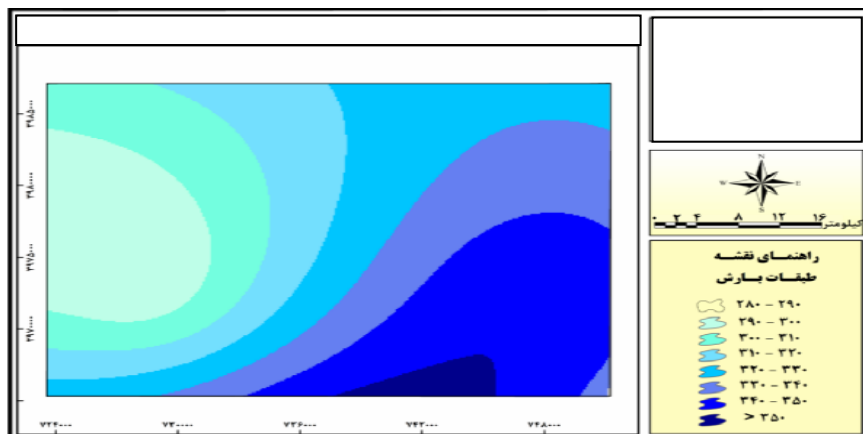
شکل (۱۱) نقشه همباران شهرستان بیجار
