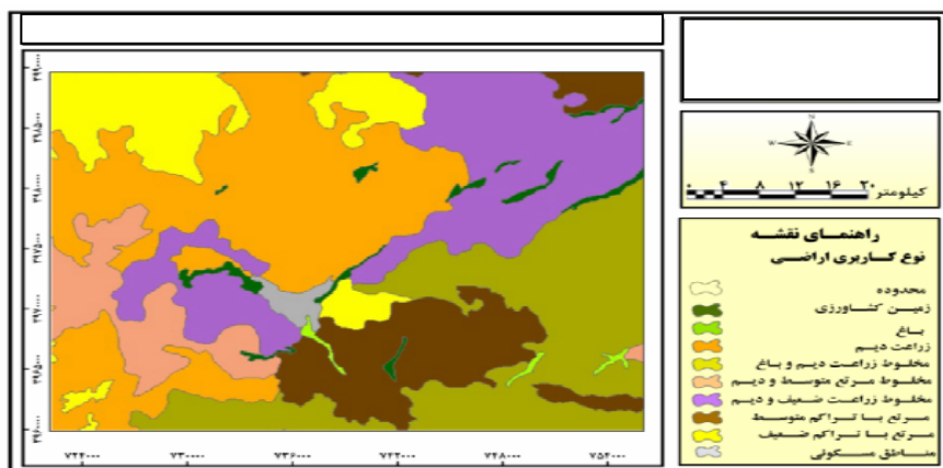
شکل (۱۲) نقشه کاربری اراضی شهرستان بیجار
