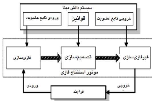
شکل ۱- ساختار اصلی سیستم‌های استنتاج فازی (کیا ۱۳۸۹).
