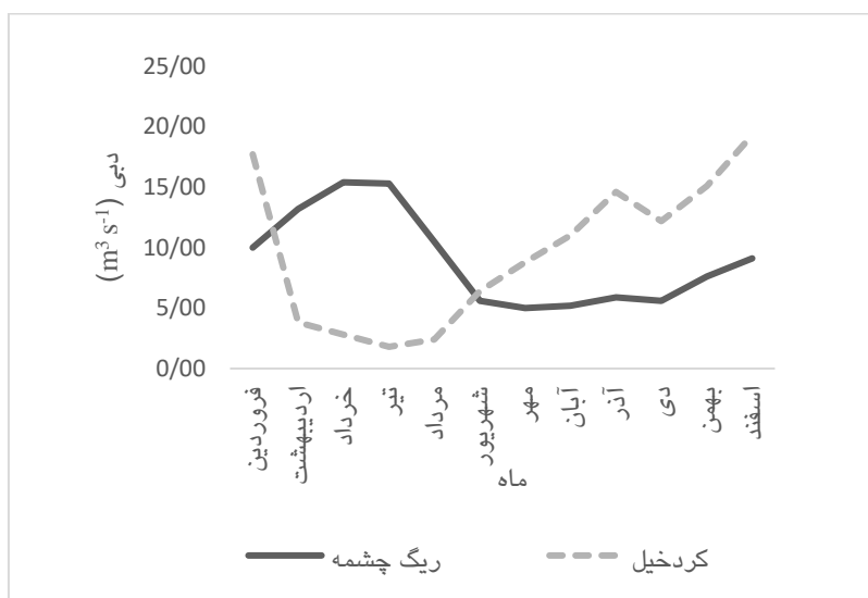
شکل ۲- تغییرات میانگین دبی روزانه در ایستگاههای ریگ چشمه و کردخیل در ماههای سال.
