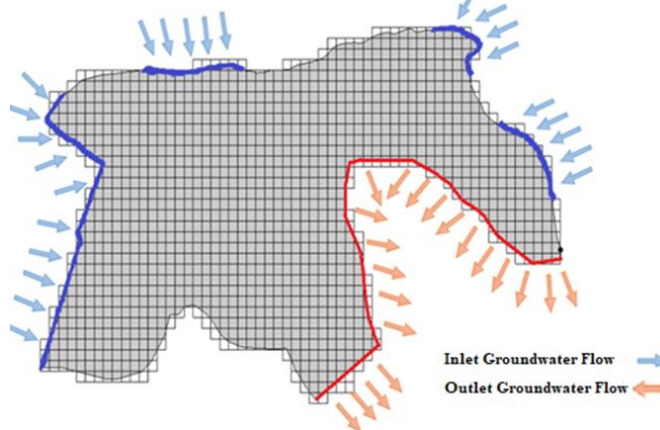
شکل ۳- جریان ورودی و خروجی آب زیرزمینی در مرز آبخوان.
