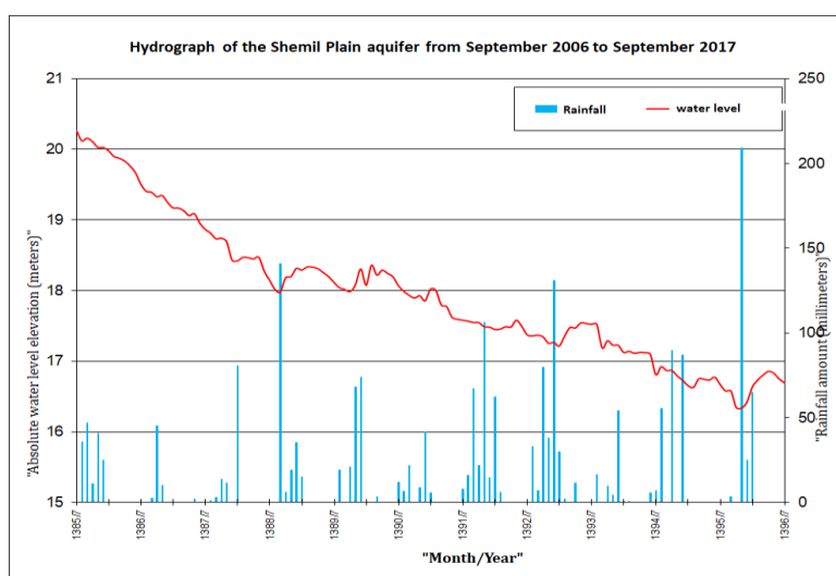
شکل ۱- هیدروگراف معرف آبخوان دشت شمیل طی سال‌های ۱۳۹۶ - ۱۳۸۵، (Iran Water Resources Management Company, 2015).
