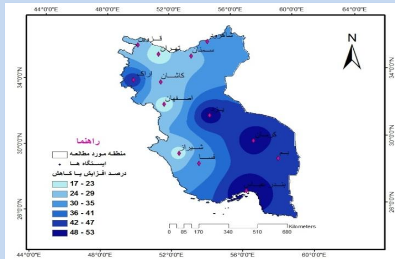
شکل 4) نقشه میزان افزایش و کاهش (%) بارش زمستانه منطقه مورد مطالعه در شرایط سرد SST دریای مدیترانه به شرایط گرمتر در پاییز
