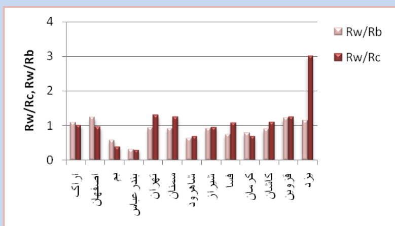
نمودار (7) نسبت میان‌ه بارش پاییزه منطقه مورد مطالعه در شرایط گرم‌تر دمای تابستانه سطح آب دریای مدیترانه به میان‌ه بارش آن در شرایط سردتر و معمول آن
