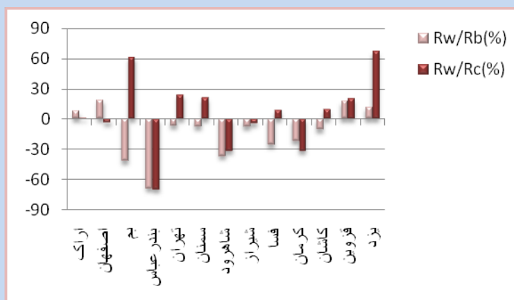
نمودار (8) میزان افزایش و کاهش (%) بارش پاییزه منطقه مورد مطالعه در شرایط گرم‌تر SST دریای مدیترانه به شرایط سردتر و معمول آن در فصل تابستان
