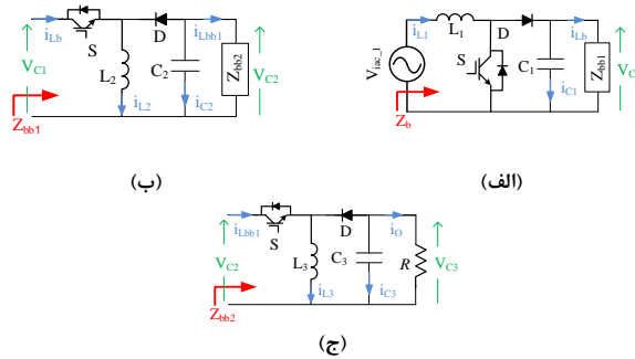
شکل ۶- مدل ac بخشهای مختلف درایور پیشنهادی و امپدانسهای ورودی آنها - الف) بوست، ب) باک-بوست اول و ج) باک-بوست دوم
