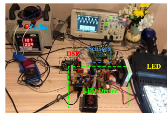
شکل ۱۰- نمونه آزمایشگاهی درایور LED پیشنهادی
