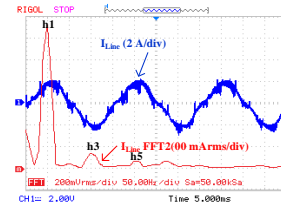
شکل ۱۲- نتایج عملی جریان در سمت ac و تبدیل فوریه آن
