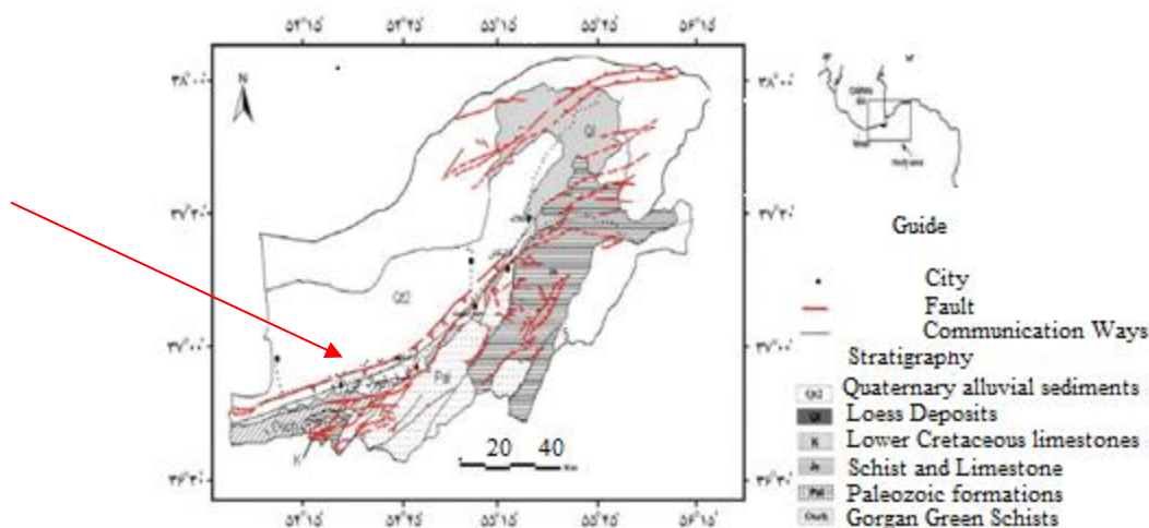
شکل (۸): نقشه زمین‌شناسی ساده شده و گسل‌های کوارتزی از گستره مورد مطالعه و پیرامون آن (با تغییراتی از صالحی و همکاران، ۲۰۱۳)
