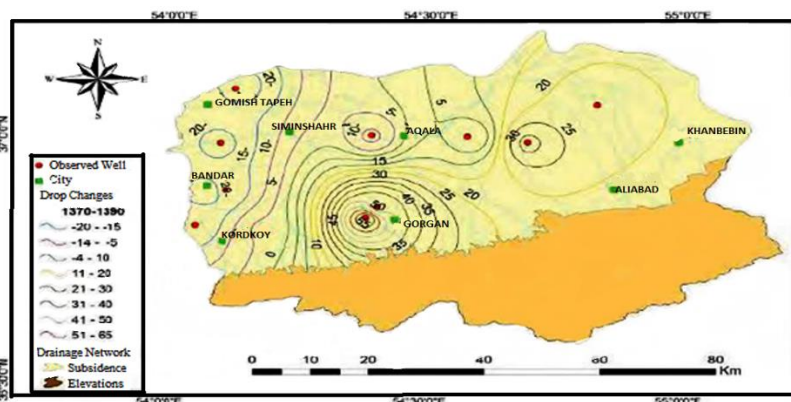
شکل (۴): تغییرات سطح آب زیرزمینی دشت گرگان (نمودار هم‌افت) (شایان و همکاران، ۲۰۱۵) Fig. 4-Groundwater level changes in Gorgan plain (drop Fig.)
