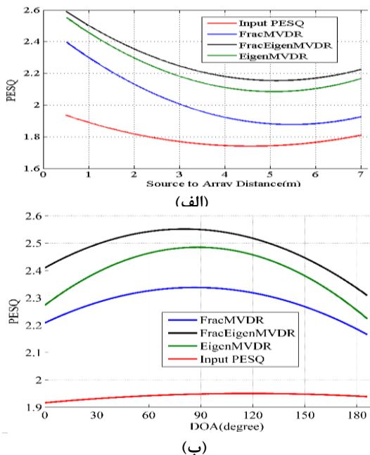
شکل ۴: کیفیت شنیداری روش‌های پیشنهادی بر حسب تغییرات: (الف) فاصله منبع تا آرایه و (ب): زاویه ورود سیگنال
