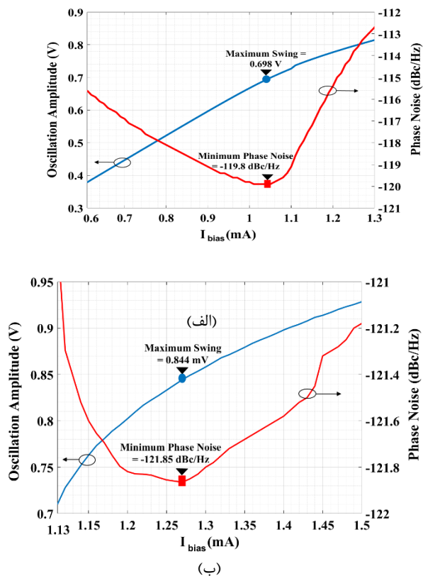
شکل ۱۱: دامنه نوسان و نویز فاز (در آفست ۱MHz از فرکانس حامل ۵GHz) بر حسب جریان بایاس برای نوسان‌ساز کنترل شده با ولتاژ (الف) متداول و (ب) پیشنهادی
