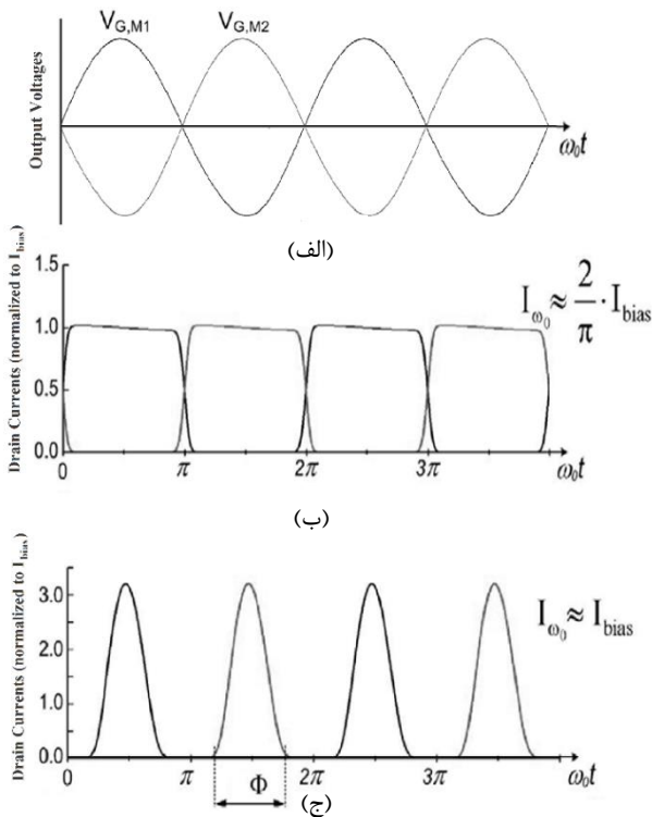
شکل ۲: (الف) ولتاژهای خروجی سینوسی نوسان‌ساز LC؛ جریان‌های گذرنده از ترانزیستورهای هسته در نوسان‌ساز LC نوع (ب) کلاس-B و (ج) کلاس-C [۵]
