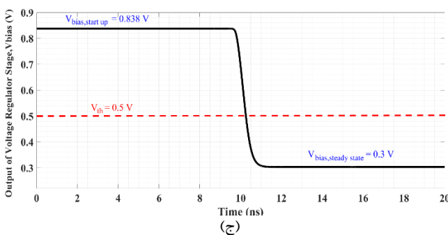
شکل ۸: شکل موج‌های گذرا در مدار تنظیم بایاس نوسان ساز پیشنهادی
