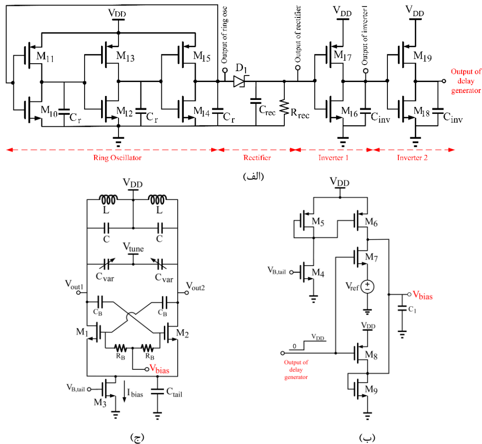
شکل ۷: شماتیک VCO کلاس-C پیشنهادی؛ (الف) طبقه تولید کننده تاخیر؛ (ب) طبقه تنظیم ولتاژ؛ (ج) هسته کلاس-C
