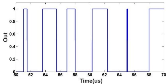
شکل ۷- نتایج شبیه‌سازی خروجی مولد اعداد شبه تصادفی پیشنهادی پیاده‌سازی شده با بلوک‌های Generator System Xilinx
