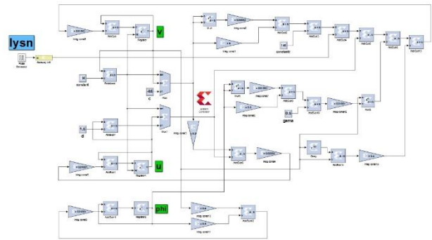
شکل ۴- پیاده‌سازی دیجیتالی نوسان‌ساز نوری پیشنهادی با استفاده از ابزار generator system Xilinx
