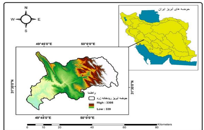
شکل (۱): مختصات و موقعیت جغرافیایی منطقه مورد مطالعه (منبع: نویسندگان)
