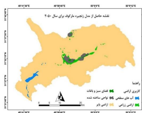
شکل (۹) - نقشه حاصل از مدل CA-Markov برای سال ۲۰۵۰
