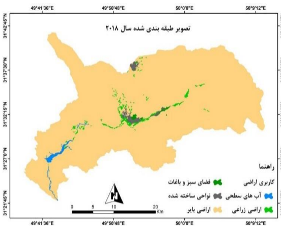
شکل (۶)- نقشه مرجع سال ۲۰۱۸ (منبع نویسندگان)
