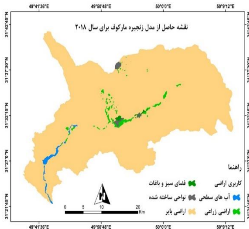
شکل (۷)- نقشه حاصل از مدل CA-Markov برای سال ۲۰۱۸ (منبع نویسندگان)
