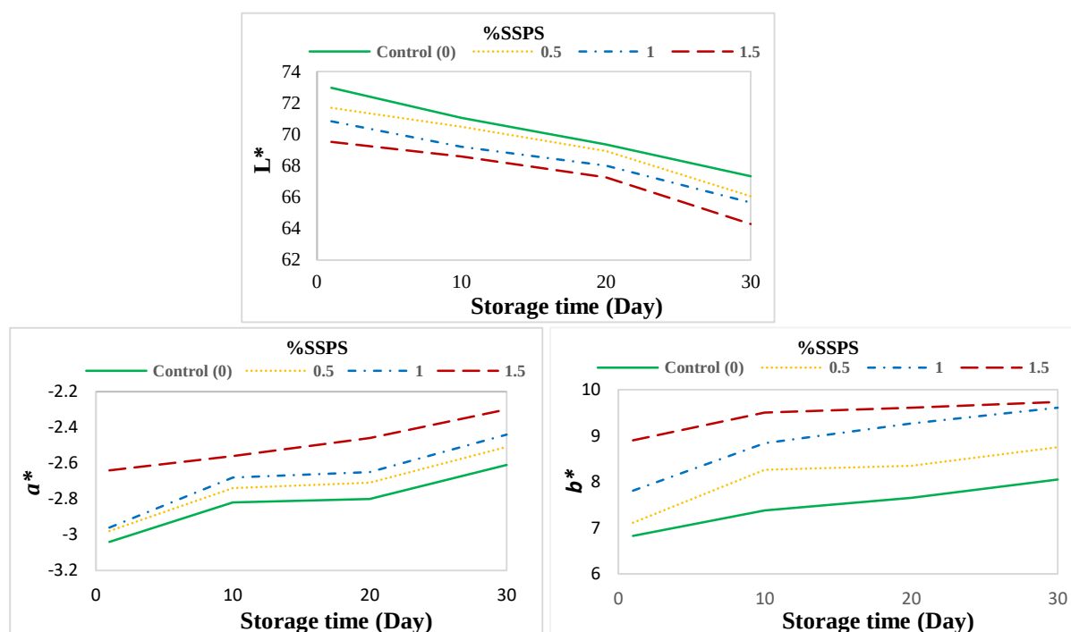
شکل ۱- تأثیر زمان و مقادیر مختلف پلی ساکارید محلول سویا (SSPS) بر پارامترهای رنگی کفیر حاصل از شیر سویا طی مدت سی روز نگهداری در ۴ درجه سلسیوس
