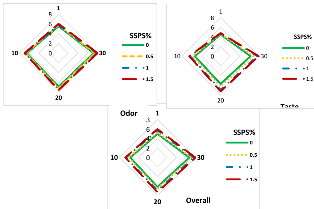
شکل ۲- تأثیر زمان و میزان پلی ساکارید محلول سویا (SSPS) بر ویژگی‌های حسی کفیر شیر شویا طی سی روز نگهداری در ۴ درجه سلسیوس
