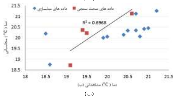
شکل ۵- میزان همبستگی دما مشاهداتی و محاسباتی در مرحله صحت‌سنجی: الف) Landsat8، ب) Sentinel2
