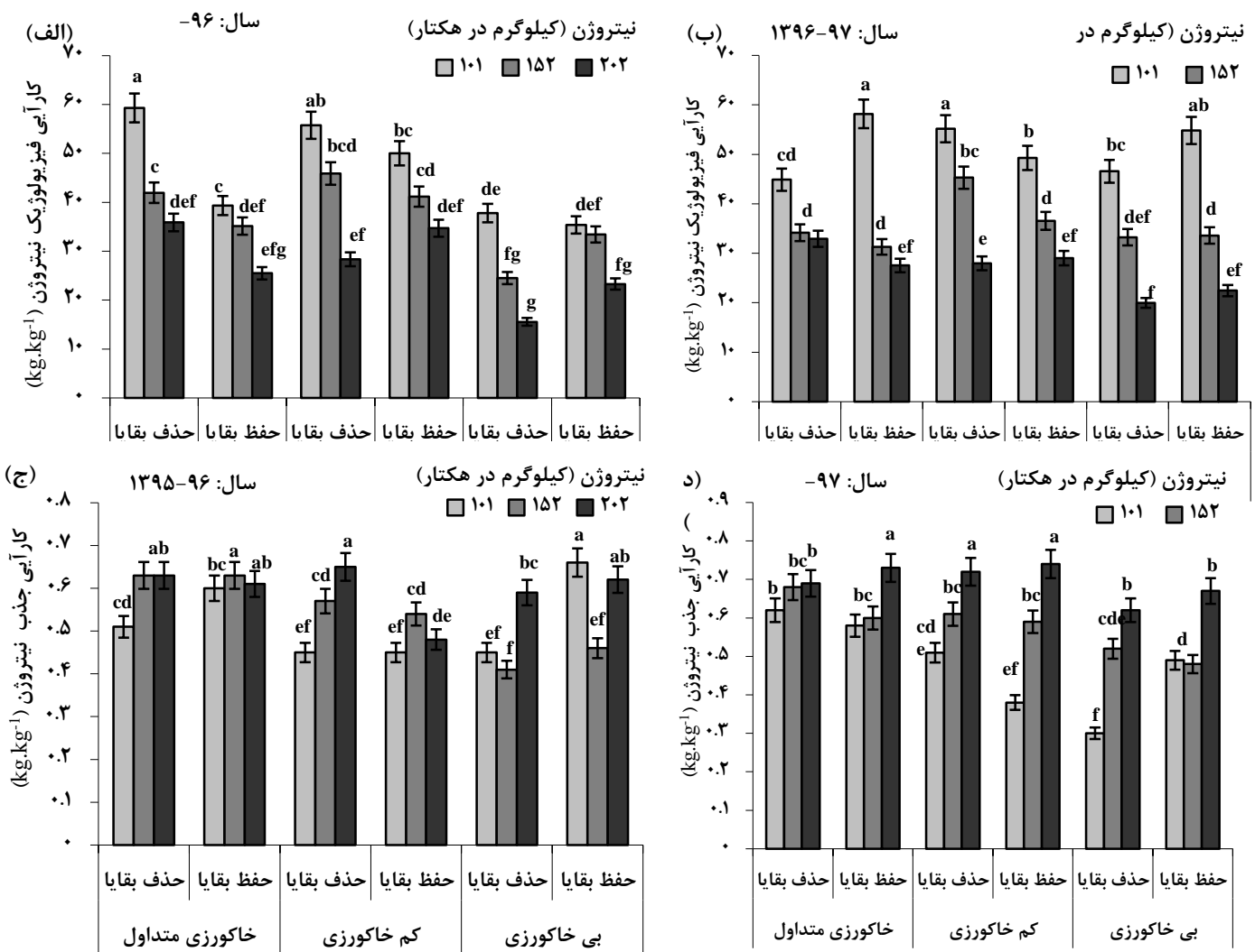
شکل ۲- اثر روش‌های خاک‌ورزی و مقادیر نیتروژن بر کارایی فیزیولوژیک و کارایی جذب نیتروژن گندم در تناوب گندم-نرت در دو سال زراعی ۱۳۹۵-۹۶ و ۱۳۹۶-۹۷ (ستون‌های با حروف مشابه بر اساس آزمون چند دامنه‌ای دانکن در سطح ۵ درصد تفاوت معنی-داری ندارند)
