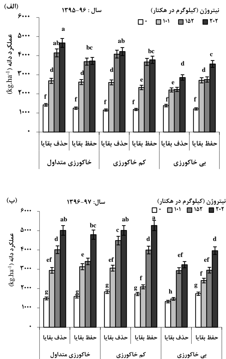
شکل ۴- اثر روش‌های خاک‌ورزی و مقادیر نیتروژن بر عملکرد دانه گندم در تناوب گندم-ذرت در دو سال زراعی ۱۳۹۵-۹۶ و
