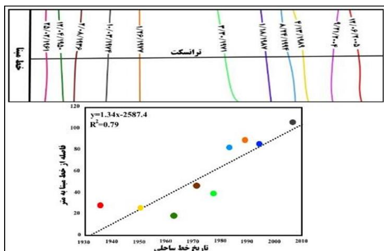
شکل (۴): نحوه محاسبه خط رگرسیون در روش LRR که در این روش تمامی سال‌ها و زمان آن‌ها در محاسبات آورده می‌شوند (هیملستوس، ۲۰۰۹).
