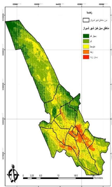
شکل (۷): نقشه ی طبقه بندی خطر مناطق سیل خیز Fig (7): Risk classification map of flood-prone areas
