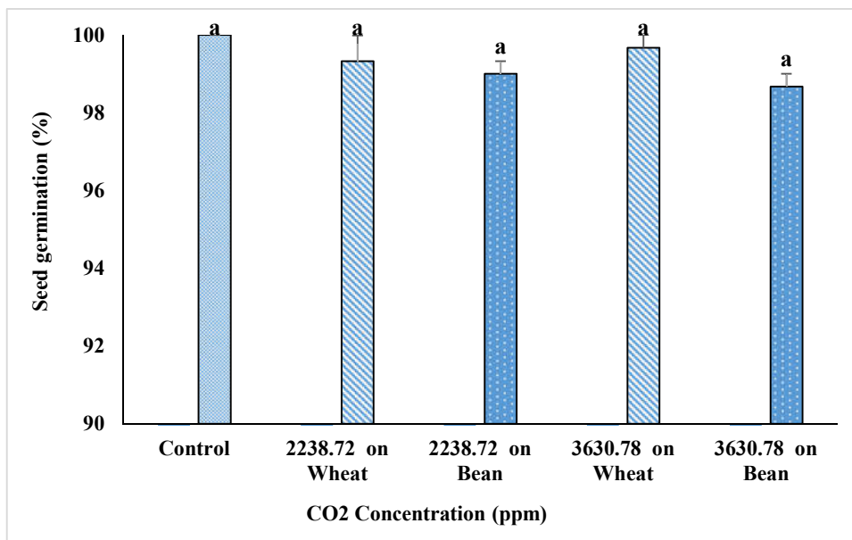
شکل ۱. اثر غلظت‌های مختلف گاز دی اکسید کربن روی جوانه‌زنی بذور لوبیا چشم بلبلی و گندم.
