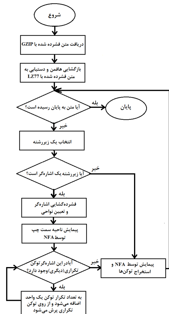
شکل ۶: روندنمای روش پیشنهادی
