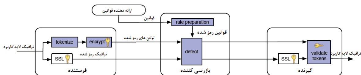
شکل ۳: شمای کلی از بازرسی محتوایی ترافیک HTTPS طبق روش Blindbox [۵]
