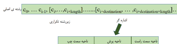
شکل ۵: نمایشی از رشته اصلی، زیر رشته تکراری، اشاره‌گر و نواحی مربوط به اشاره‌گر
