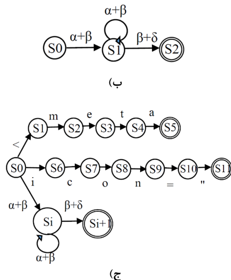
شکل ۷: مراحل طراحی ماشین حالت NFA (الف) مثال کوچکی از طراحی DFA برای پذیرش تگ‌ها و مشخصه‌ها (ب) طراحی NFA برای پذیرش توکن‌هایی با طول نامعلوم (ج) ماشین حالت NFA نهایی برای پذیرش توکن‌های معنادار
