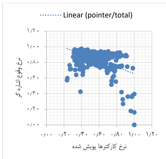
شکل ۱۰: نسبت نرخ وقوع اشاره گر به نرخ کاراکترهای پوشش شده به ازای هر ۵۰۰ فایل
