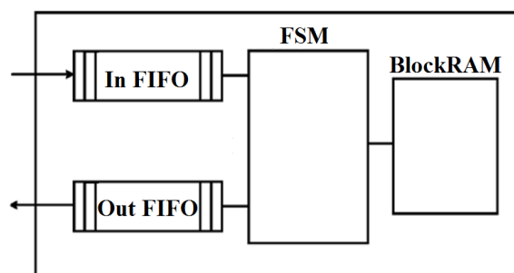
شکل ۱۲: بلاک دیاگرام سخت‌افزار پیشنهادی
