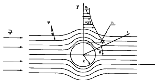
شکل 2- خطوط جریان اطراف سیلندر استوانه‌ای
