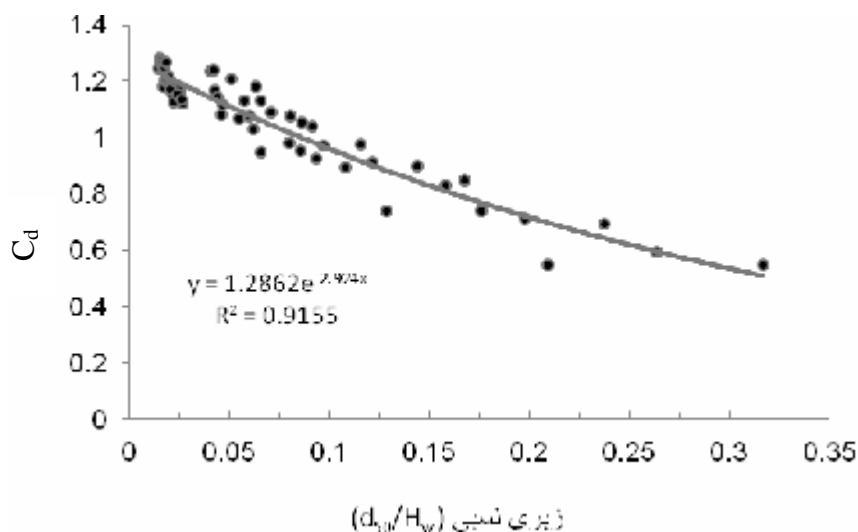
شکل 6- تغییرات ضریب تخلیه در مقابل زبری نسبی ( \frac{D_{50}}{H_w} )
