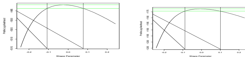
شکل ۴- نمودارهای نیمرخ لگاریتم درست‌نمایی پارامتر شکل بارش حدی (راست: ابعلی، چپ: مهرآباد).
