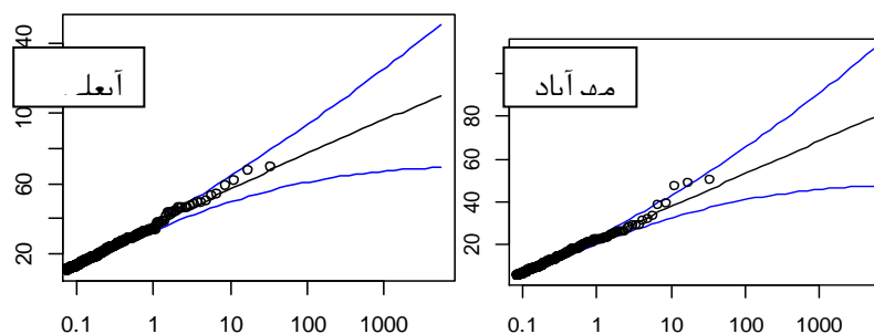
شکل ۵- منحنی‌های رشد بارش حدی با فاصله اطمینان ۹۵٪ در دوره ۲۰۱۶-۱۹۸۳. (نقاط مقادیر مشاهداتی، منحنی‌ها مقادیر برآورد شده با تابع GPD و خطوط اطراف، باند اطمینان را نشان می‌دهند).
