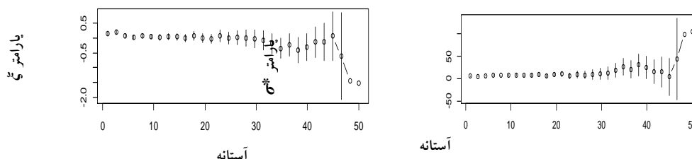
شکل ۳- نمودارهای MBC برای حداکثر بارش روزانه ایستگاه آبعلی (۱۹۸۳-۲۰۱۶).
