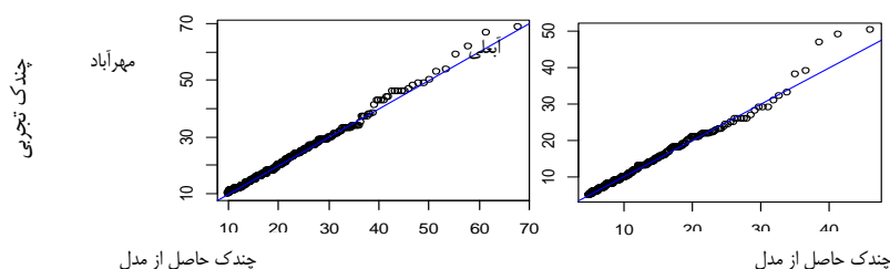
شکل ۶- نمودارهای Q-Q پس از برازش مدل POT به رویداد حدی بارش در مهرآباد در دوره ۲۰۱۶-۱۹۸۳.
