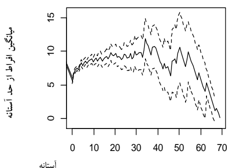
شکل ۲- نمودارهای MRL برای حداکثر بارش روزانه ایستگاه آبعلی (۱۹۸۳-۲۰۱۶).
