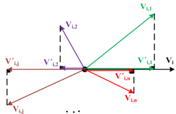
شکل ۴: نمایش برداری بردارهای ولتاژ تشکیل دهنده بردار ولتاژ باس مورد بررسی به همراه تصویر آن‌ها بر بردار ولتاژ باس مورد بررسی
