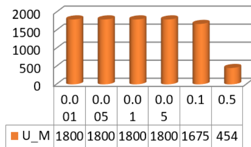
شکل ۸: تعداد نمونه‌های انتخاب شده از پایگاه‌داده U_M
