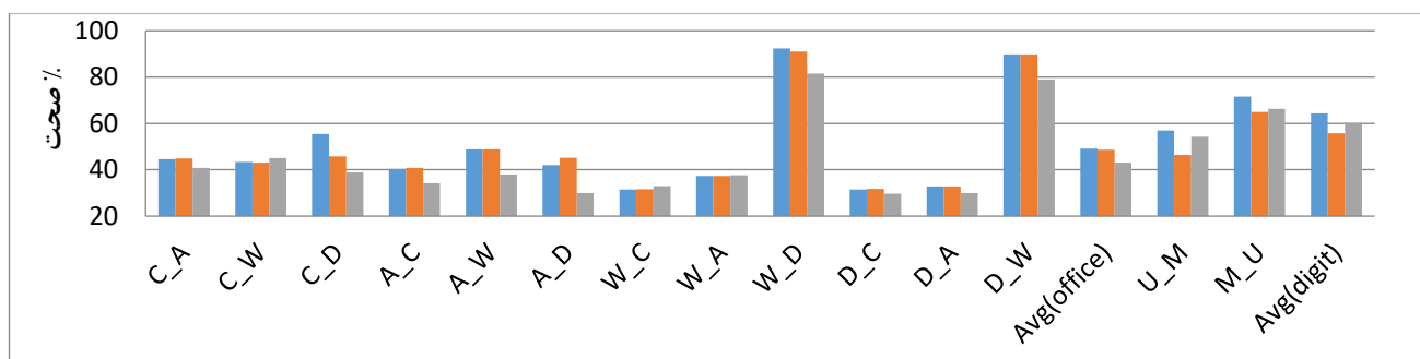
شکل ۱۰: مقایسه کارایی روش پیشنهادی (SCDA) در صورت عدم استفاده از تطبیق زیرفضا ( SCDA^{subspace} ) و عدم استفاده از اختلاف توزیع شرطی ( SCDA^{conditional} ) (نمایش بهتر به صورت رنگی)
