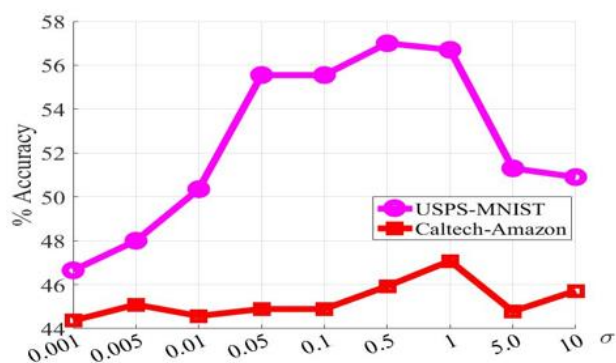
شکل ۷: ارزیابی صحت پایگاه داده های C_A و U_M با مقادیر مختلف پارامتر \delta ، ضریب MMD
