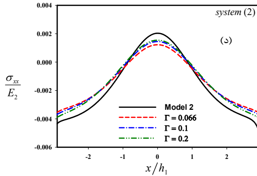
شکل ۱۳- توزیع تنش داخل صفحه بر روی فصل مشترک لایه هدفمند با الف و ج- پوشش سخت و ب و د- بستر همگن به ازای مقادیر مختلف نسبت سفتی ( \eta = 0.5 , \frac{E_x}{E_y} = 3 , P = 10\text{KN} , R=100\text{mm} , \nu = 0.3 , x=1 ( E_{0x} = E_1 = 116.36 \text{ Gpa} , E_2 = 20 \text{ Gpa} , \nu = 0.3 ).
