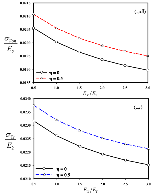
شکل ۷- تغییرات بیشینه تنش‌های الف- فون میسر ب- ترسکا در بستر به ازای مقادیر مختلف نسبت مدول الاستیسیته ( \theta = 0 ) E_2 = 20 \text{ Gpa} , \nu = 0.3 , h_2/h_1 = 1 , P = 10\text{KN} , R=100\text{mm} , 0 (E_{0X} = E_1 = 116.36 \text{ Gpa} , 20 \text{ Gpa} )
