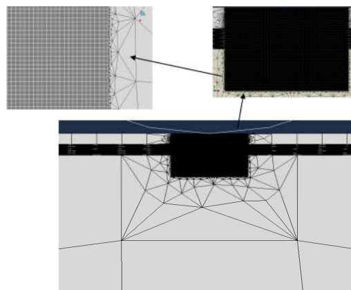
شکل ۲- شبکه بندی مسئله مورد بررسی
