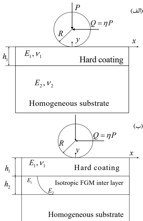
شکل ۶- الف- مدل ۱ متشکل از یک پوشش همگن ایزوتروپ و یک بستر همگن ایزوتروپ می‌باشد ب- مدل ۲ متشکل از یک پوشش همگن ایزوتروپ یک میان لایه هدفمند ایزوتروپیک و یک بستر همگن ایزوتروپ است.
