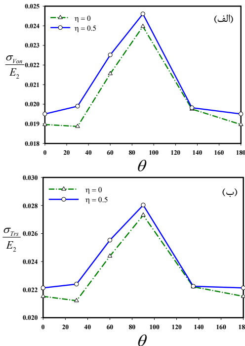
شکل ۸- بیشینه تنش‌های الف- فون میسز ب- ترسکا در بستر به ازای مقادیر مختلف زاویه جهت‌های اصلی ارتوتروپی لایه هدفمند E_2 = \nu = 0.3, \frac{h_2}{h_1} = 1, \frac{E_x}{E_y} = 3, R=100mm, P = 10KN ( E_{0x} = E_1 = 116.36 \text{ Gpa}, E_2 = 20 \text{ Gpa} )
