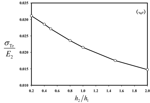
شکل ۹- بیشینه تنش‌های الف- فون میسز ب- ترسکا در بستر به ازای مقادیر مختلف ضخامت لایه هدفمند ارتوتروپیک ( R=100mm, \eta = \nu = 0.3, h_1 = 5mm, \frac{E_x}{E_y} = 3, P = 10KN, 0.5 ) ( E_{0x} = E_1 = 116.36 \text{ Gpa}, E_2 = 20 \text{ Gpa} )
